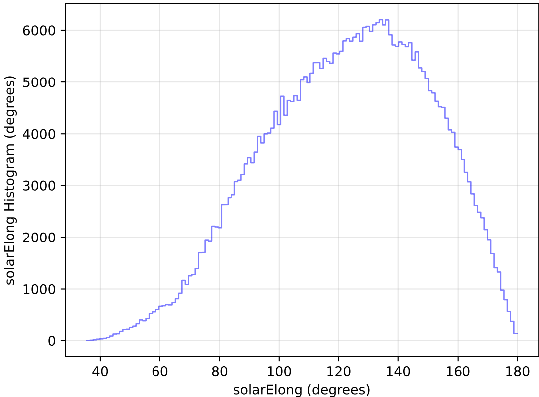
weather_cloudso16v3.4_10yrs WFD y band: solarElong Histogram
