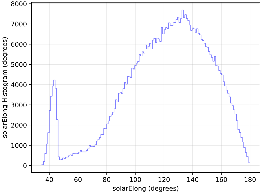
weather_cloudso16v3.4_10yrs WFD i band: solarElong Histogram
