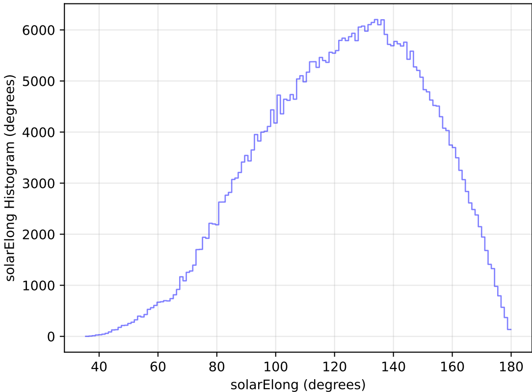
weather_cloudso16v3.4_10yrs All sky y band: solarElong Histogram
