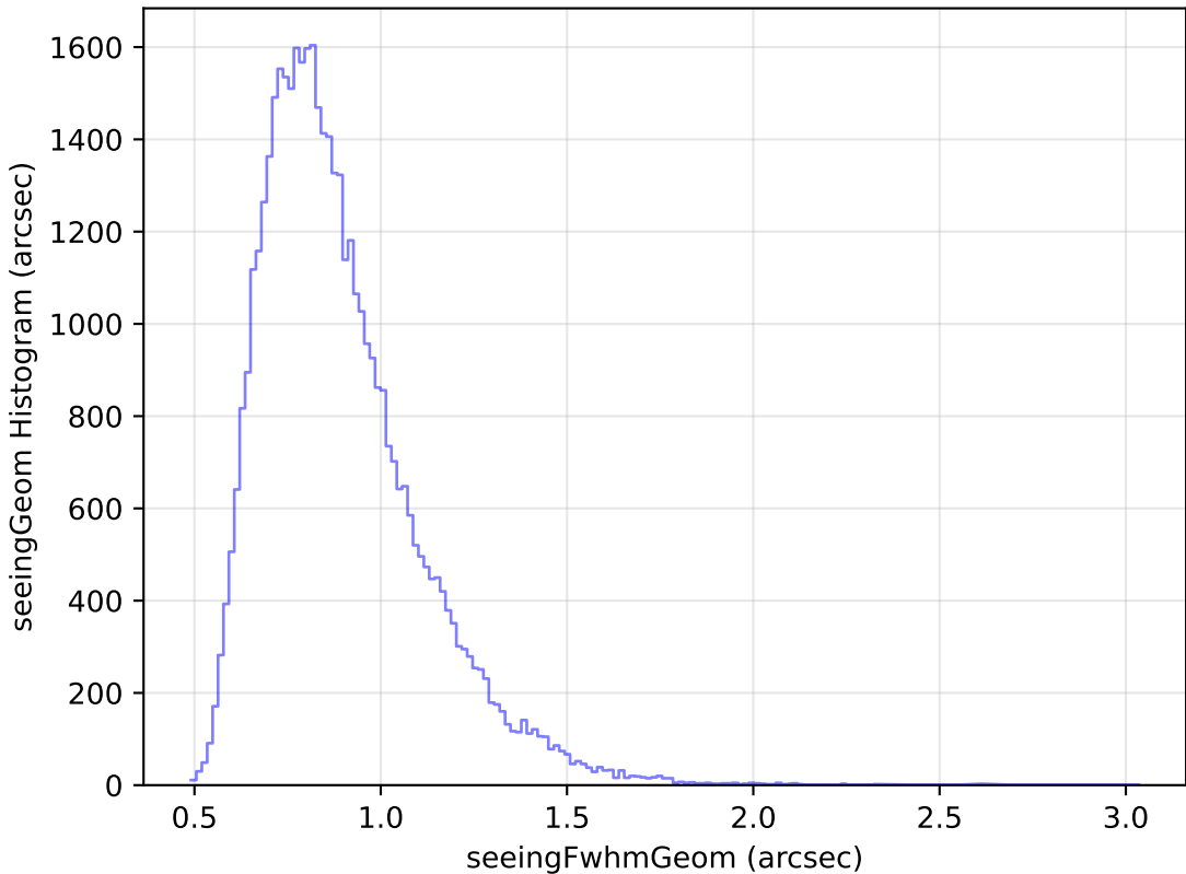
weather_cloudso16v3.4_10yrs Yr 1 y band: seeingGeom Histogram
