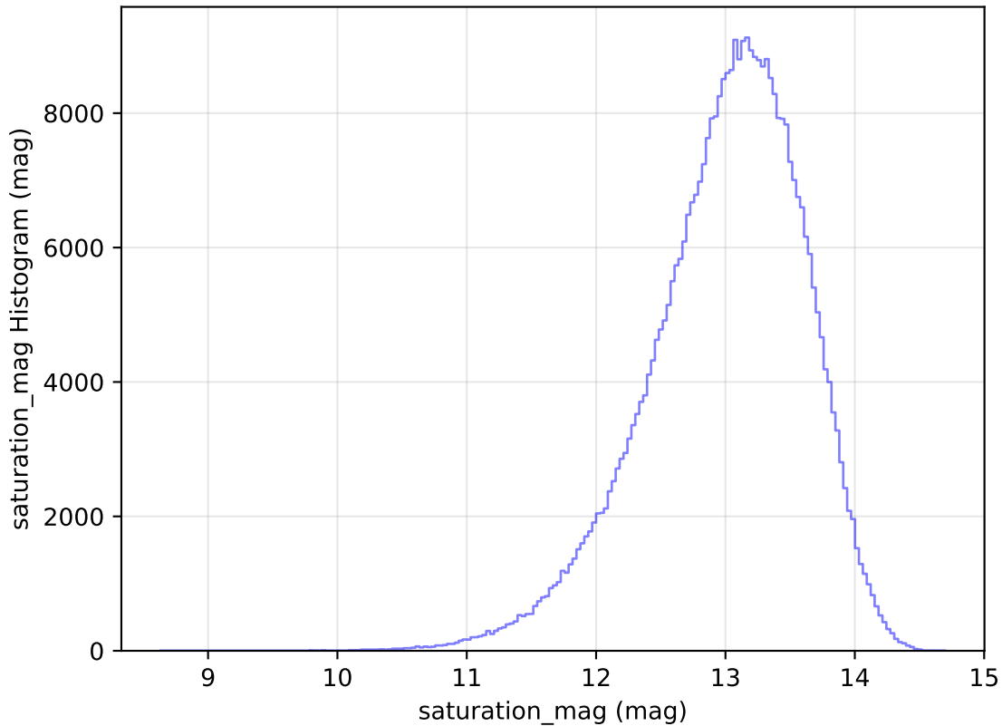
weather_cloudso16v3.4_10yrs WFD y band: saturation_mag Histogram
