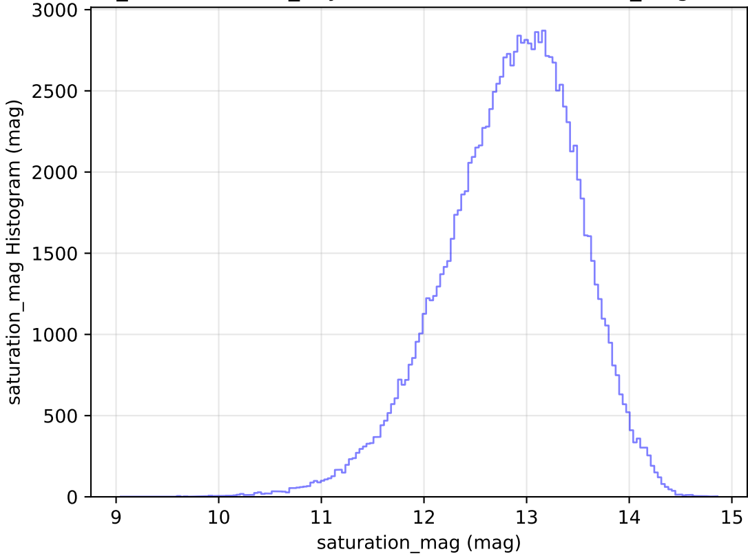
weather_cloudso16v3.4_10yrs WFD u band: saturation_mag Histogram
