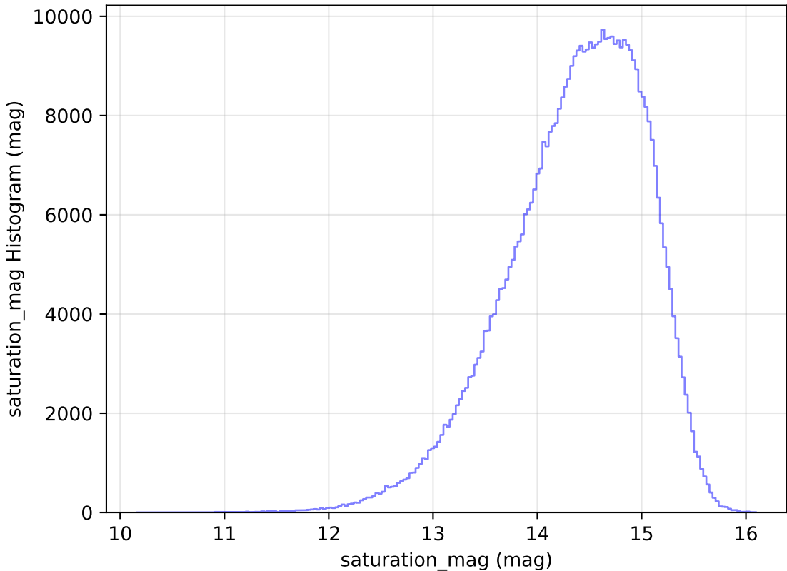
weather_cloudso16v3.4_10yrs WFD i band: saturation_mag Histogram
