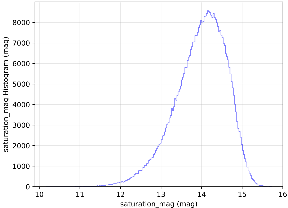
weather_cloudso16v3.4_10yrs All sky z band: saturation_mag Histogram
