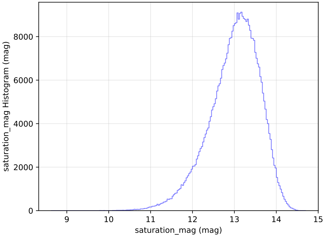
weather_cloudso16v3.4_10yrs All sky y band: saturation_mag Histogram
