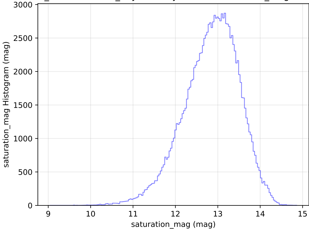
weather_cloudso16v3.4_10yrs All sky u band: saturation_mag Histogram
