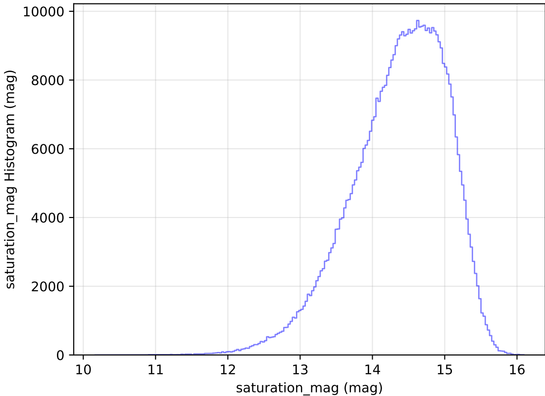
weather_cloudso16v3.4_10yrs All sky i band: saturation_mag Histogram
