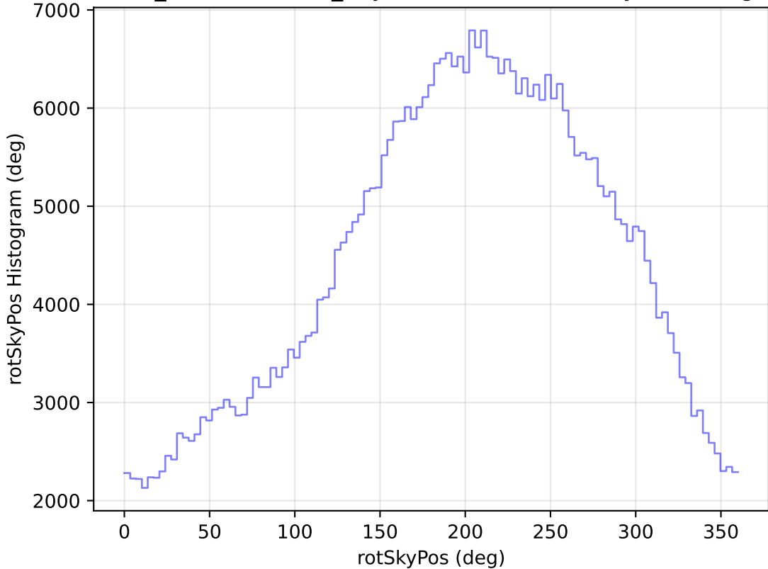
weather_cloudso16v3.4_10yrs WFD z band: rotSkyPos Histogram
