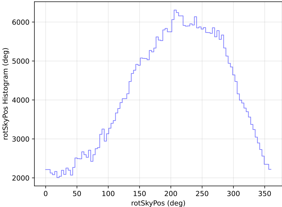
weather_cloudso16v3.4_10yrs WFD y band: rotSkyPos Histogram
