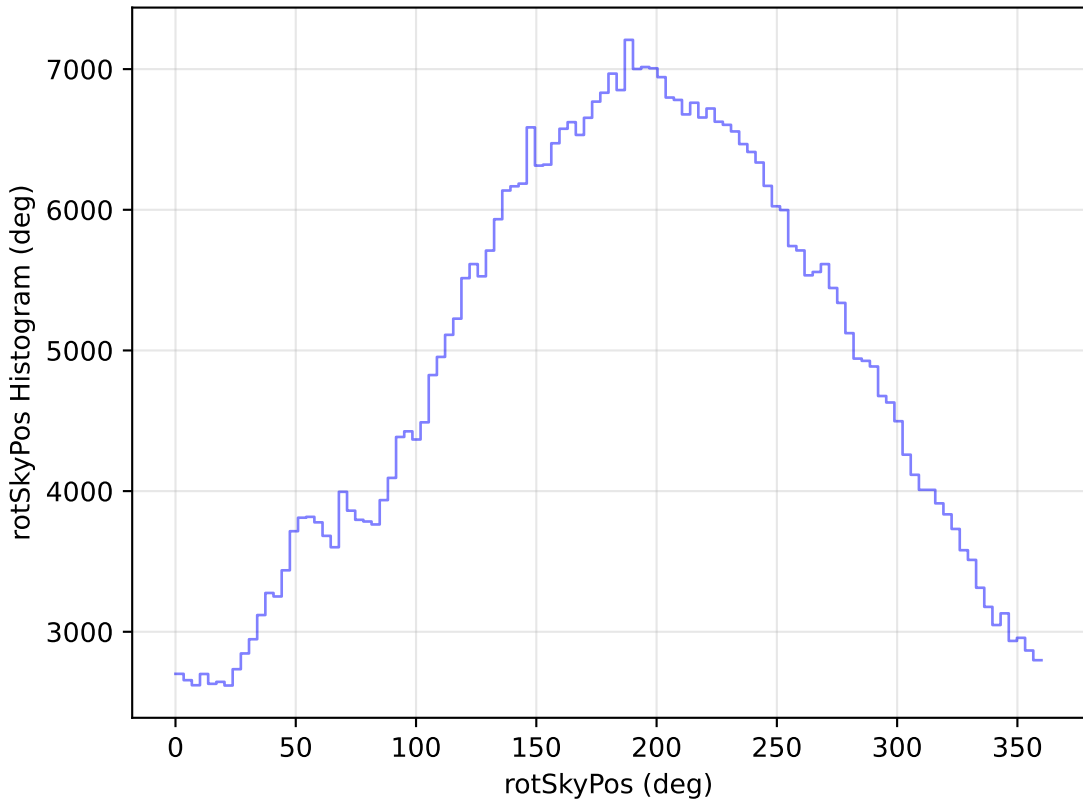
weather_cloudso16v3.4_10yrs WFD r band: rotSkyPos Histogram
