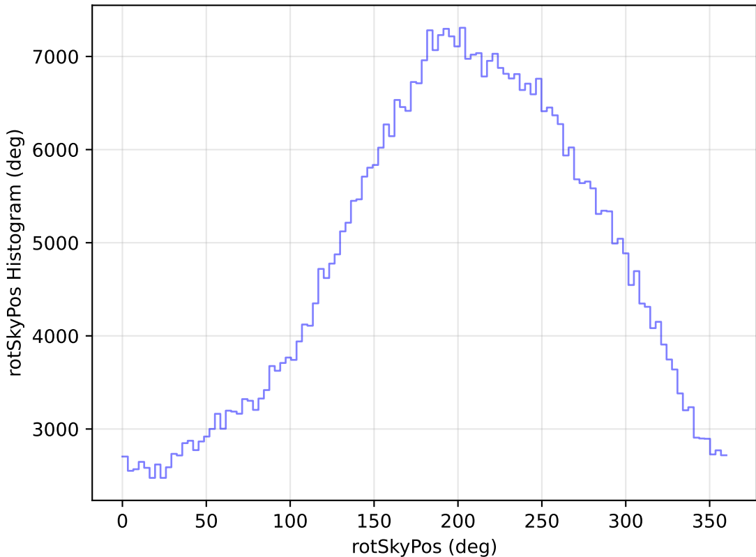
weather_cloudso16v3.4_10yrs WFD i band: rotSkyPos Histogram
