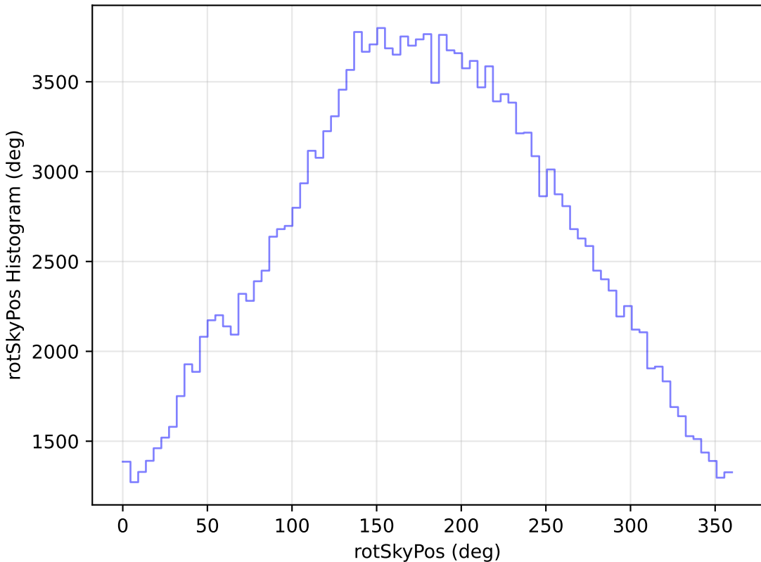
weather_cloudso16v3.4_10yrs WFD g band: rotSkyPos Histogram
