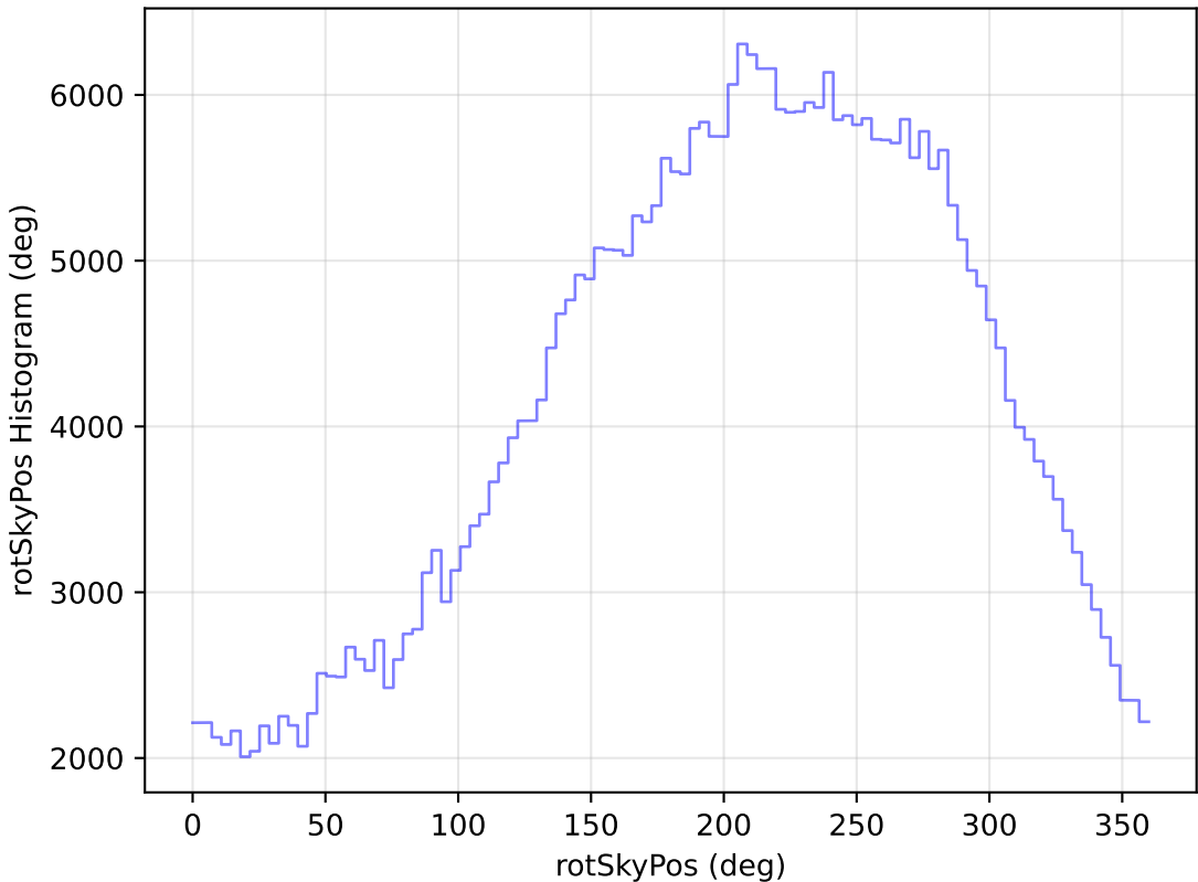
weather_cloudso16v3.4_10yrs All sky y band: rotSkyPos Histogram
