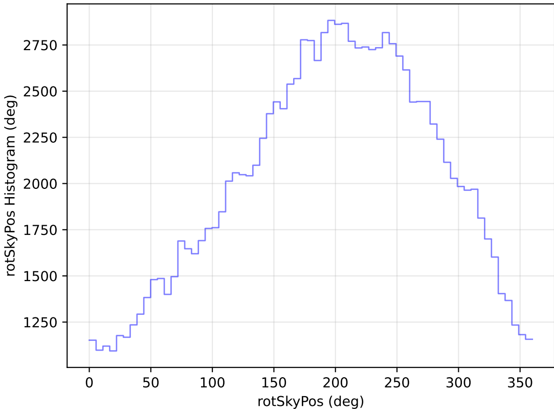
weather_cloudso16v3.4_10yrs All sky u band: rotSkyPos Histogram
