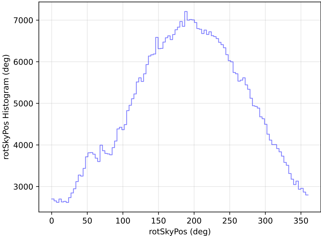
weather_cloudso16v3.4_10yrs All sky r band: rotSkyPos Histogram
