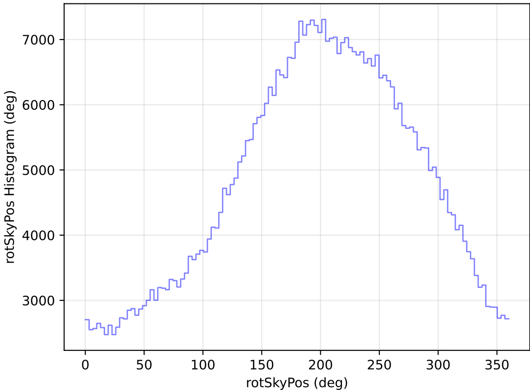
weather_cloudso16v3.4_10yrs All sky i band: rotSkyPos Histogram
