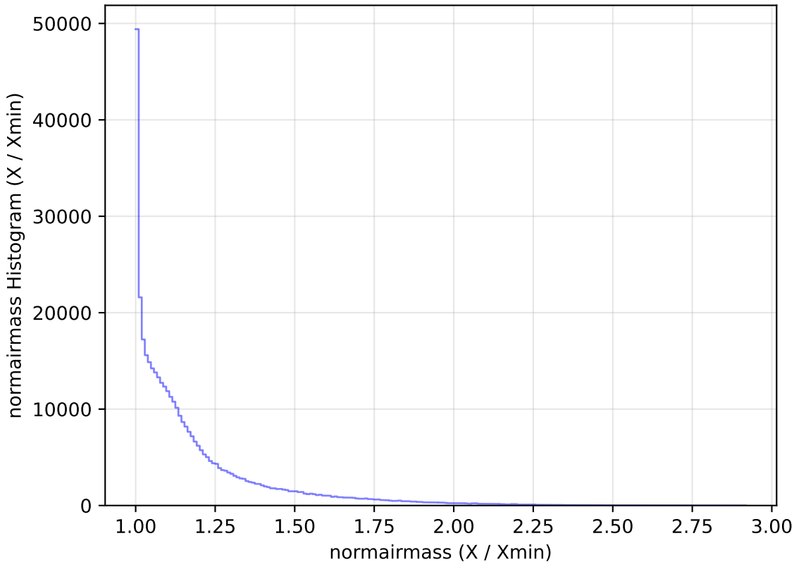
weather_cloudso16v3.4_10yrs All sky y band: normairmass Histogram
