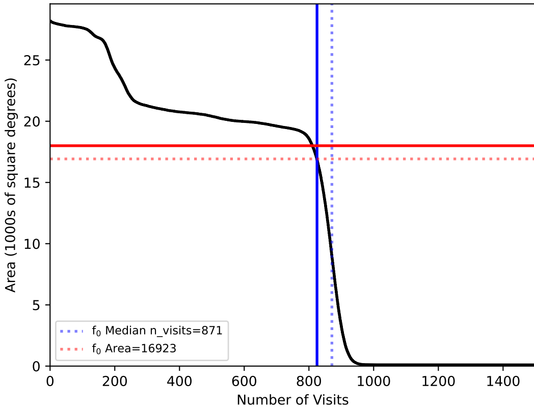
weather_cloudso16v3.4_10yrs All sky: f0
