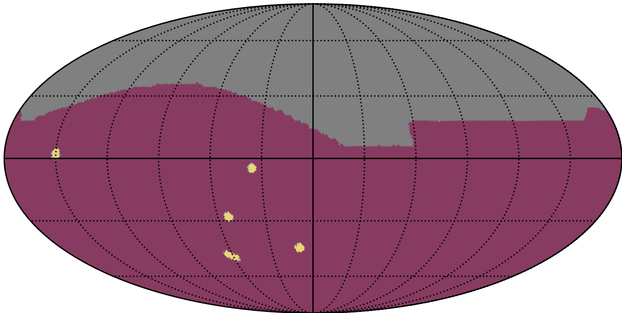
weather_cloudso16v3.4_10yrs All sky: NumberOfQuickRevisits
