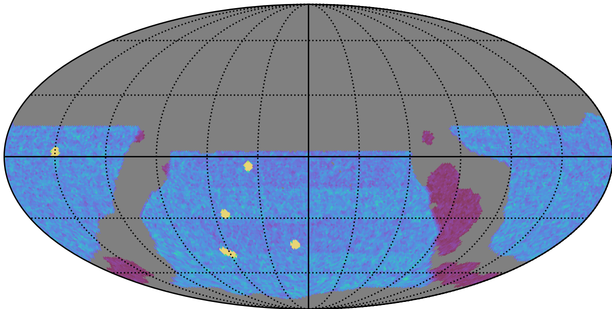
weather_cloudso16v3.4_10yrs WFD y band: NVisits
