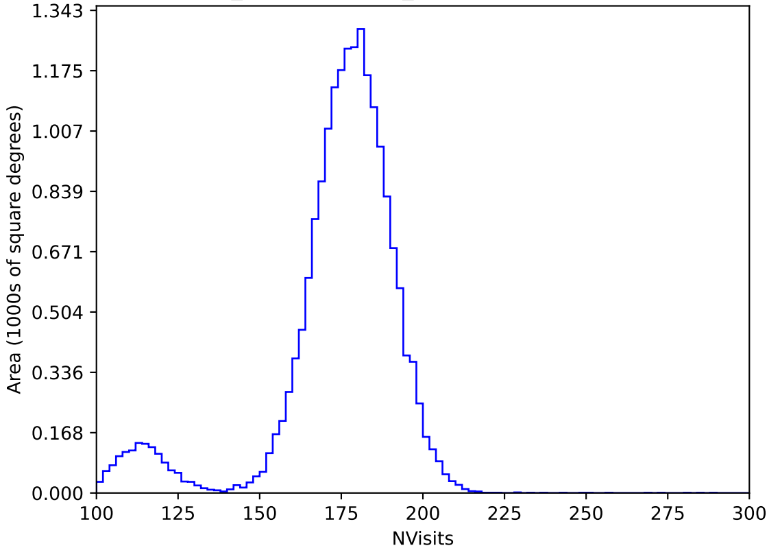
weather_cloudso16v3.4_10yrs WFD y band: NVisits
