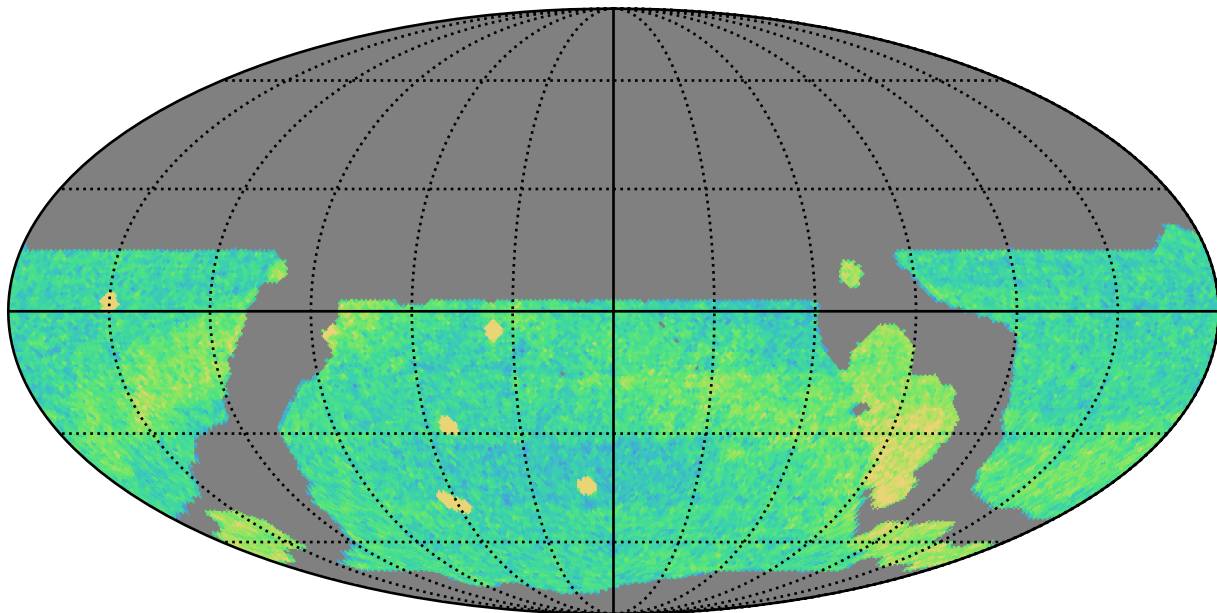
weather_cloudso16v3.4_10yrs WFD r band: NVisits
