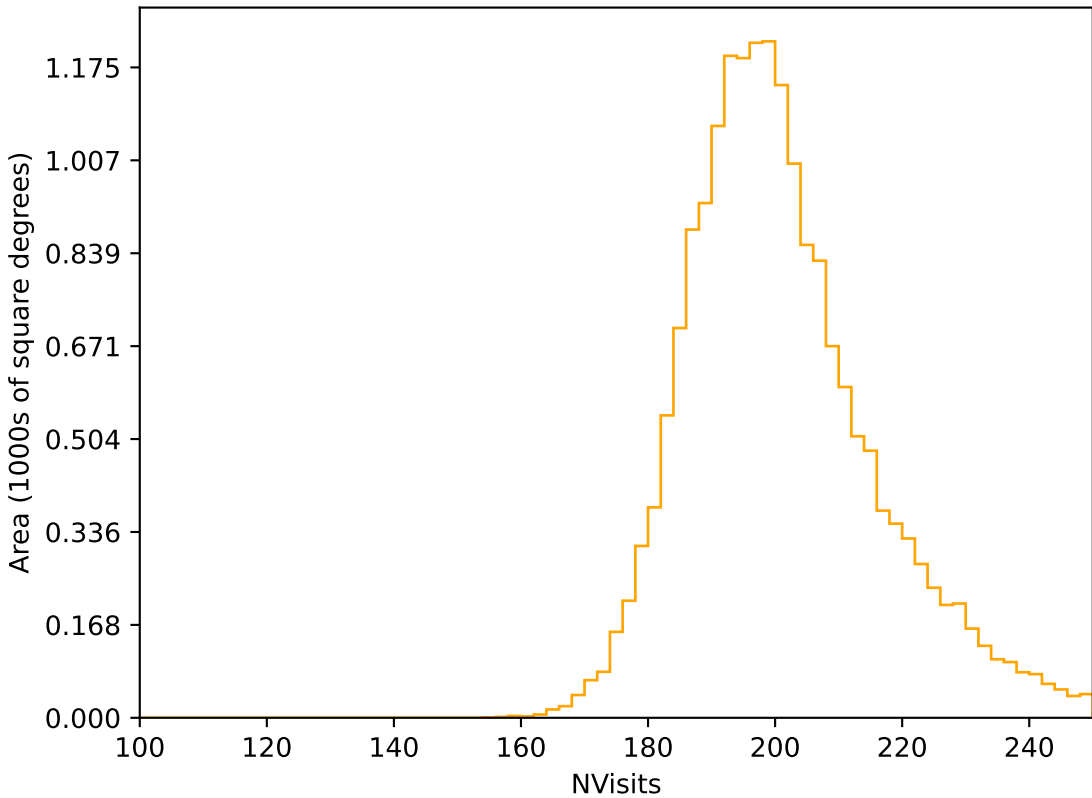
weather_cloudso16v3.4_10yrs WFD r band: NVisits
