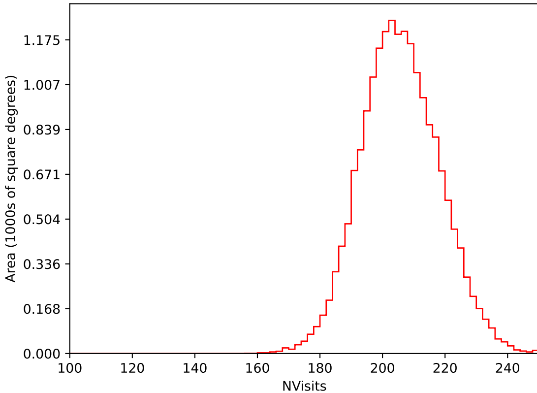
weather_cloudso16v3.4_10yrs WFD i band: NVisits
