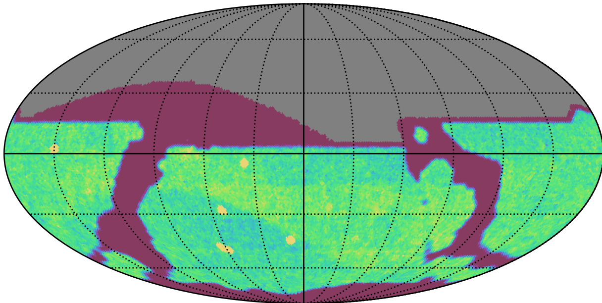
weather_cloudso16v3.4_10yrs All sky i band: NVisits
