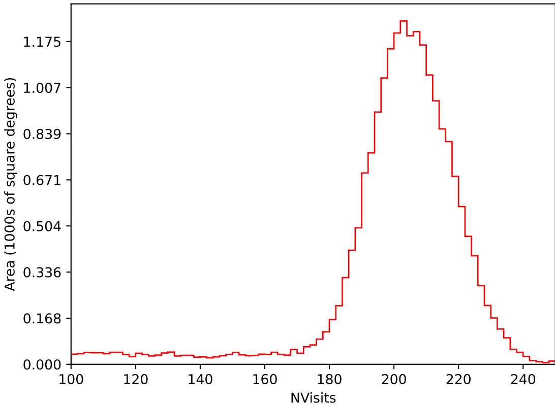
weather_cloudso16v3.4_10yrs All sky i band: NVisits
