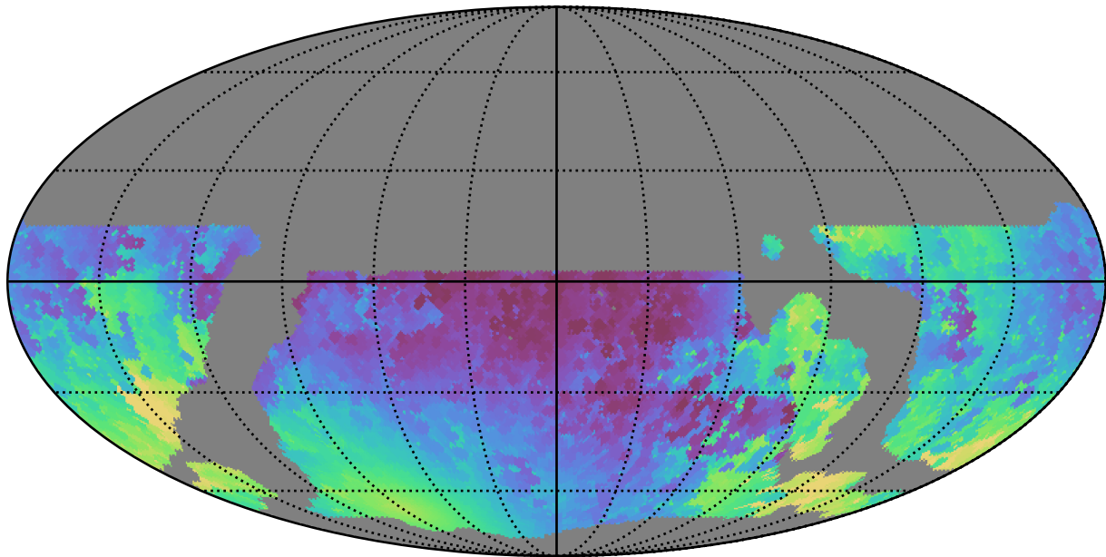
weather_cloudso16v3.4_10yrs WFD y band: Min solarElong
