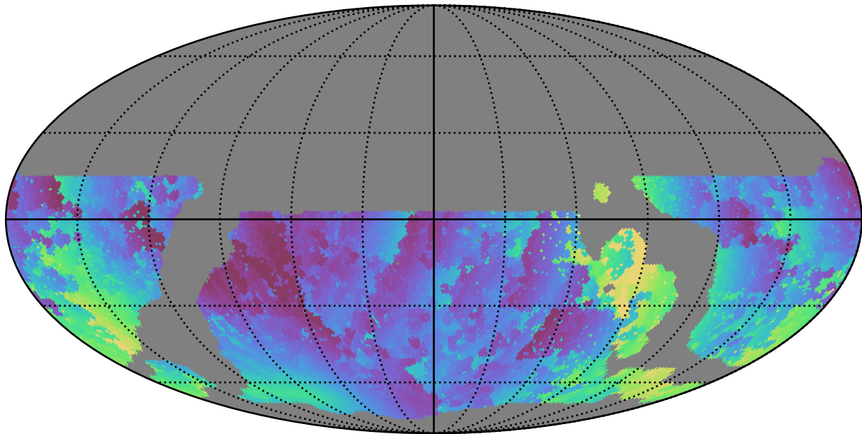
weather_cloudso16v3.4_10yrs WFD u band: Min solarElong
