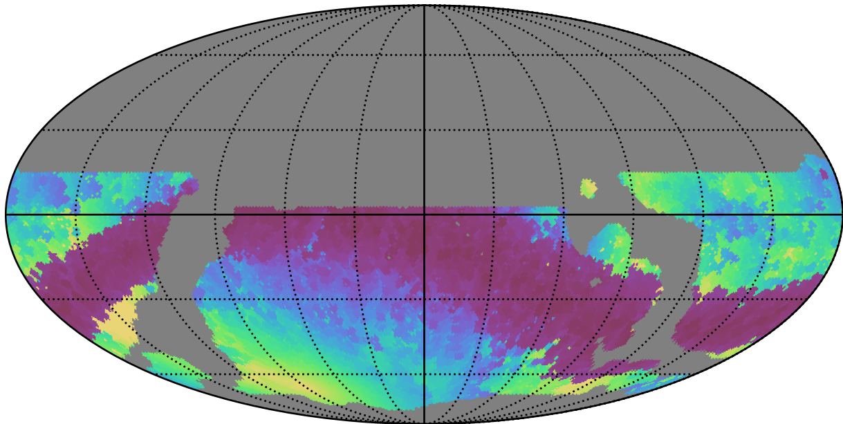
weather_cloudso16v3.4_10yrs WFD r band: Min solarElong
