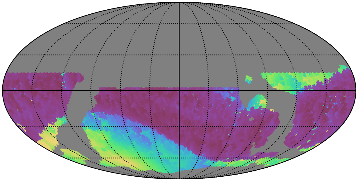
weather_cloudso16v3.4_10yrs WFD i band: Min solarElong
