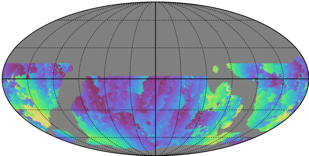
weather_cloudso16v3.4_10yrs WFD g band: Min solarElong
