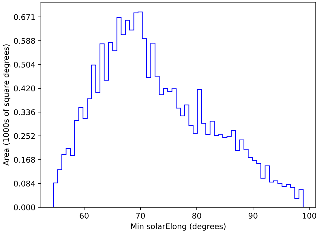
weather_cloudso16v3.4_10yrs WFD g band: Min solarElong
