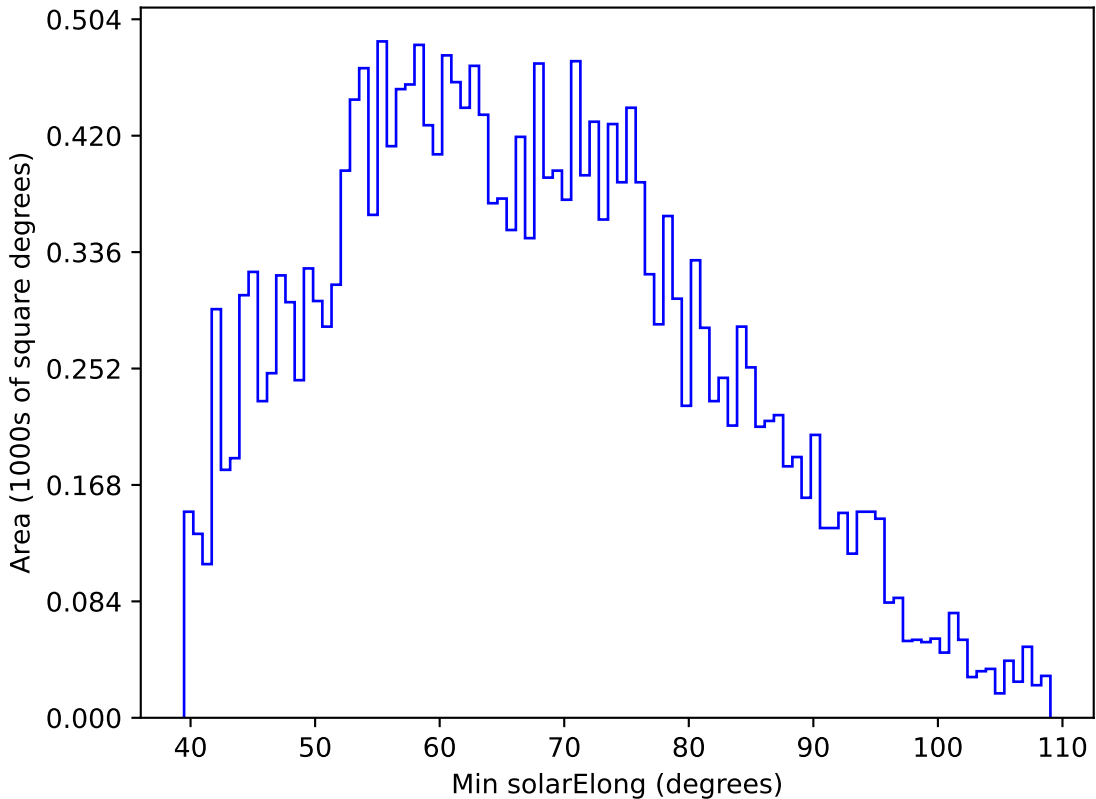
weather_cloudso16v3.4_10yrs All sky y band: Min solarElong
