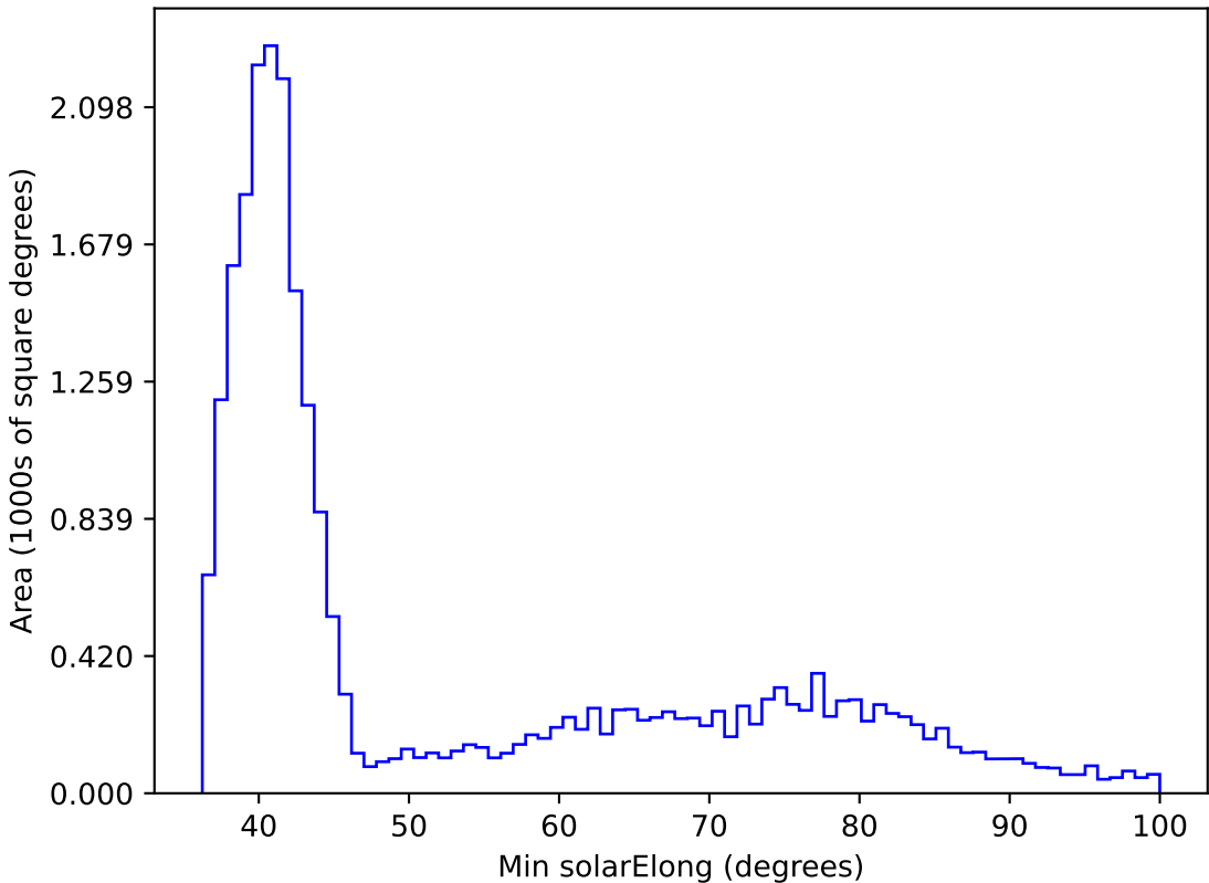
weather_cloudso16v3.4_10yrs All sky i band: Min solarElong
