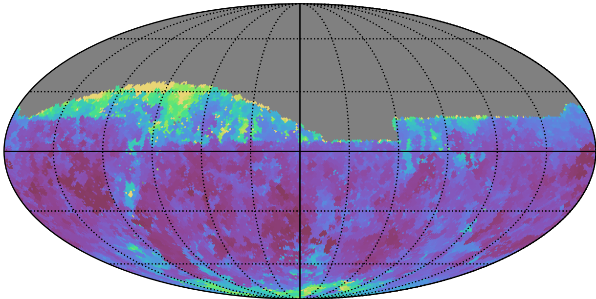
weather_cloudso16v3.4_10yrs Yr 1 z band: Min seeingGeom
