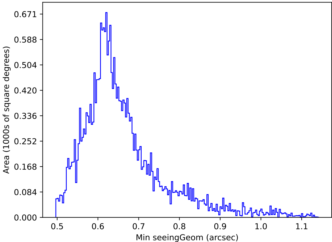
weather_cloudso16v3.4_10yrs Yr 1 z band: Min seeingGeom
