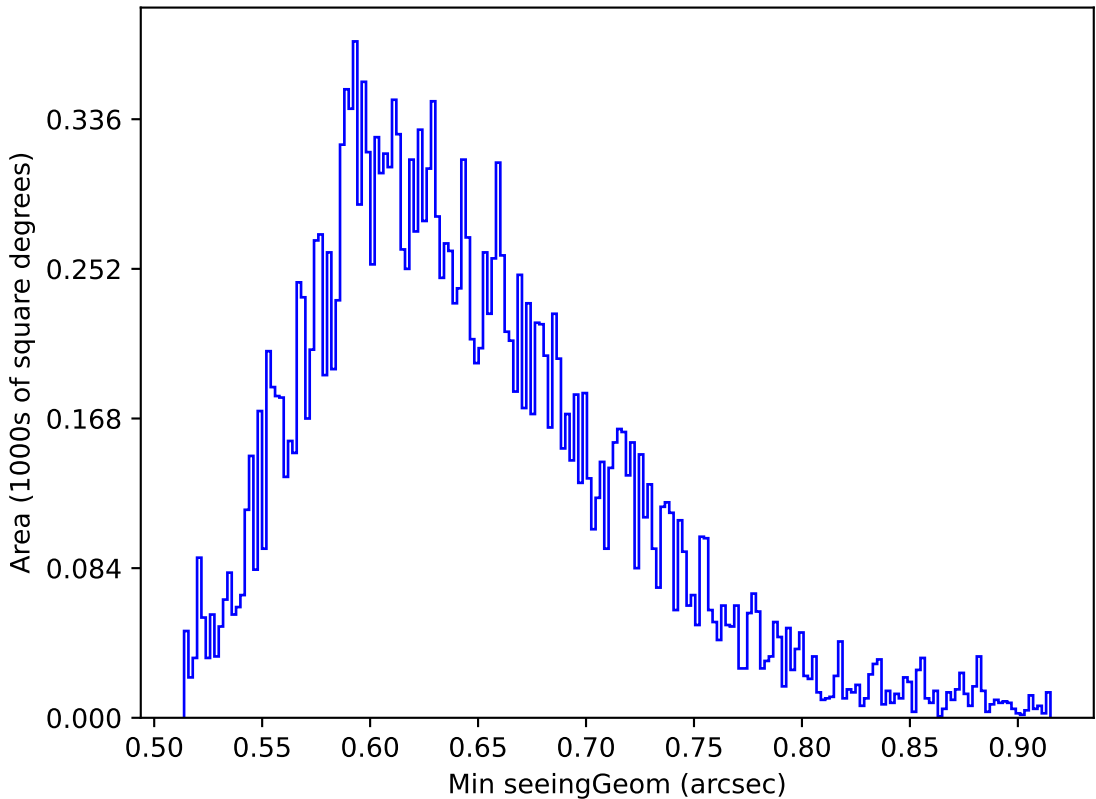
weather_cloudso16v3.4_10yrs Yr 1 y band: Min seeingGeom
