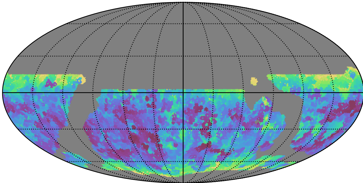
weather_cloudso16v3.4_10yrs WFD y band: Min seeingEff
