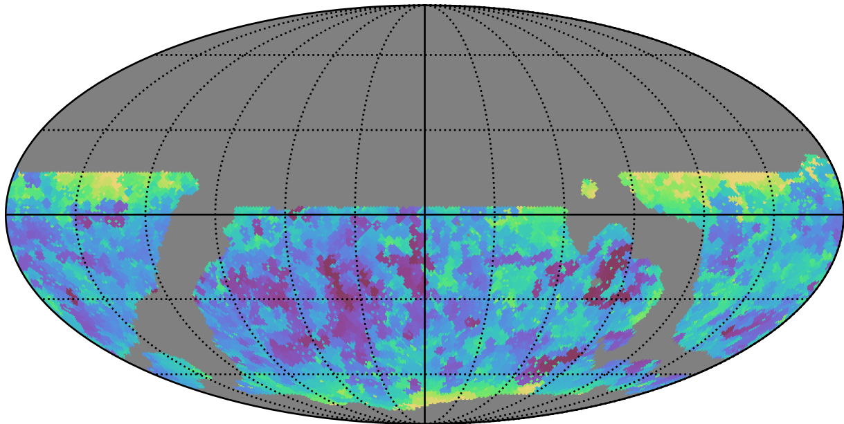
weather_cloudso16v3.4_10yrs WFD i band: Min seeingEff
