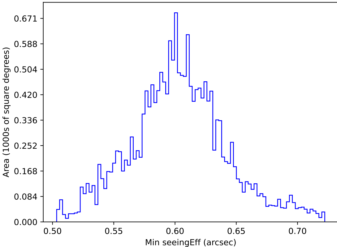
weather_cloudso16v3.4_10yrs WFD i band: Min seeingEff
