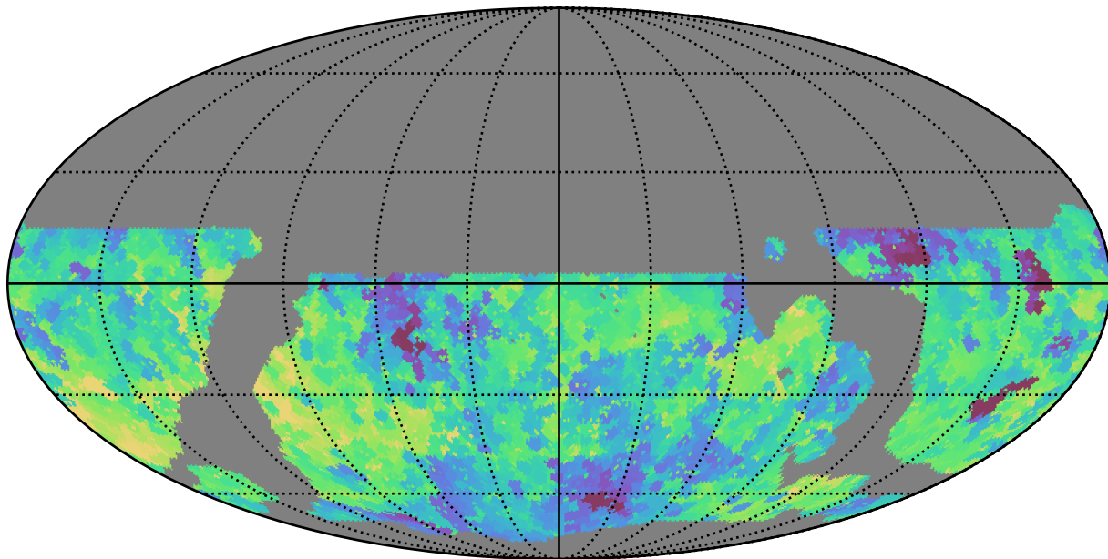
weather_cloudso16v3.4_10yrs WFD z band: Min saturation_mag
