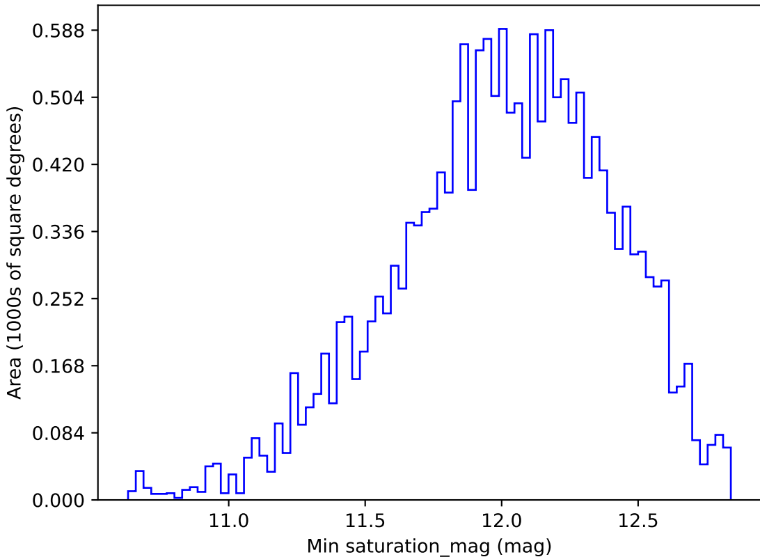
weather_cloudso16v3.4_10yrs WFD z band: Min saturation_mag
