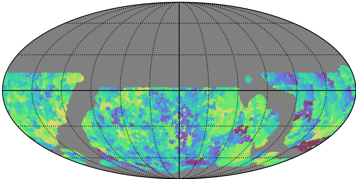
weather_cloudso16v3.4_10yrs WFD y band: Min saturation_mag
