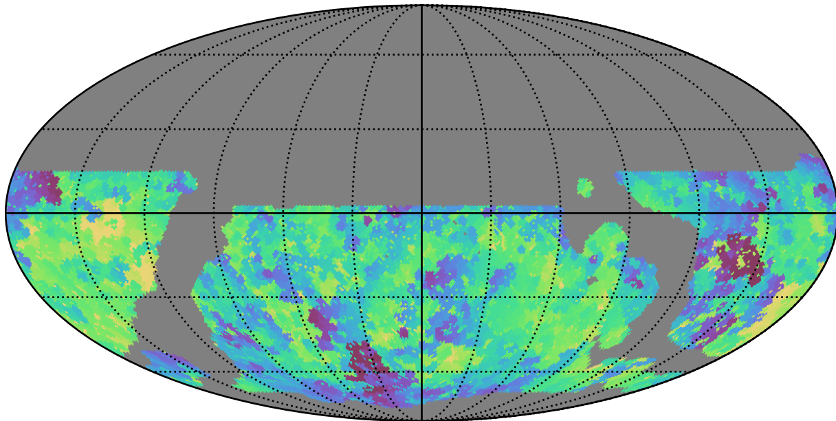
weather_cloudso16v3.4_10yrs WFD u band: Min saturation_mag
