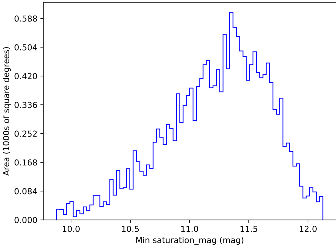
weather_cloudso16v3.4_10yrs WFD u band: Min saturation_mag
