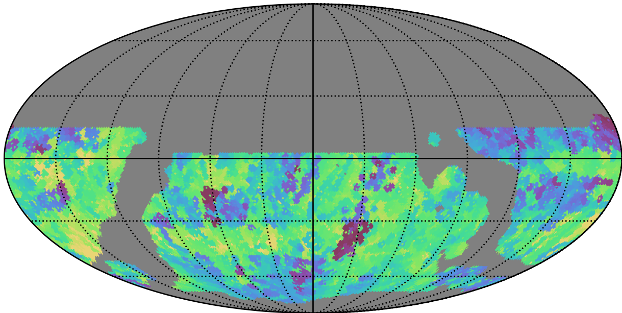
weather_cloudso16v3.4_10yrs WFD r band: Min saturation_mag
